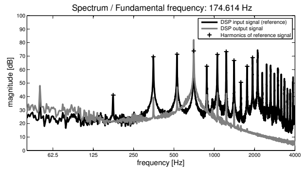
Abbildung 3: Betragsspektrum des Eingangs- und Ausgangssignals des DSPs
