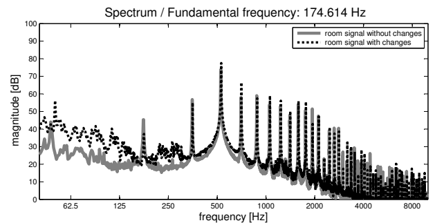
Abbildung 4: Raumspektrum vor und nach der FIR-Filterung für eine Erhöhung der 4. Harmonischen um +10 dB
