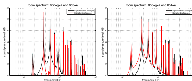
Abbildung 5: Beispiele für die Änderung des Spektrums bei Beeinflussung des Grundtons.
