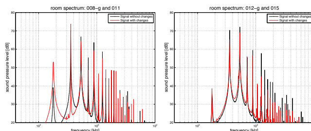
Abbildung 6: Beispiele für die Änderung des Spektrums bei Beeinflussung mehrerer Obertöne.
