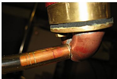
Abbildung 4: Schalleinleitung am Stiefelrohr.
