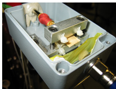
Abbildung 2: Künstlicher Anbläser.
